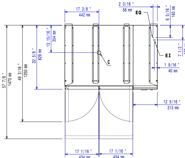
Boven aanzicht
