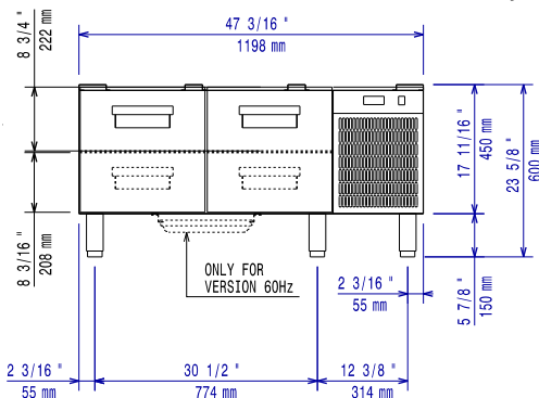
Zij aanzicht
